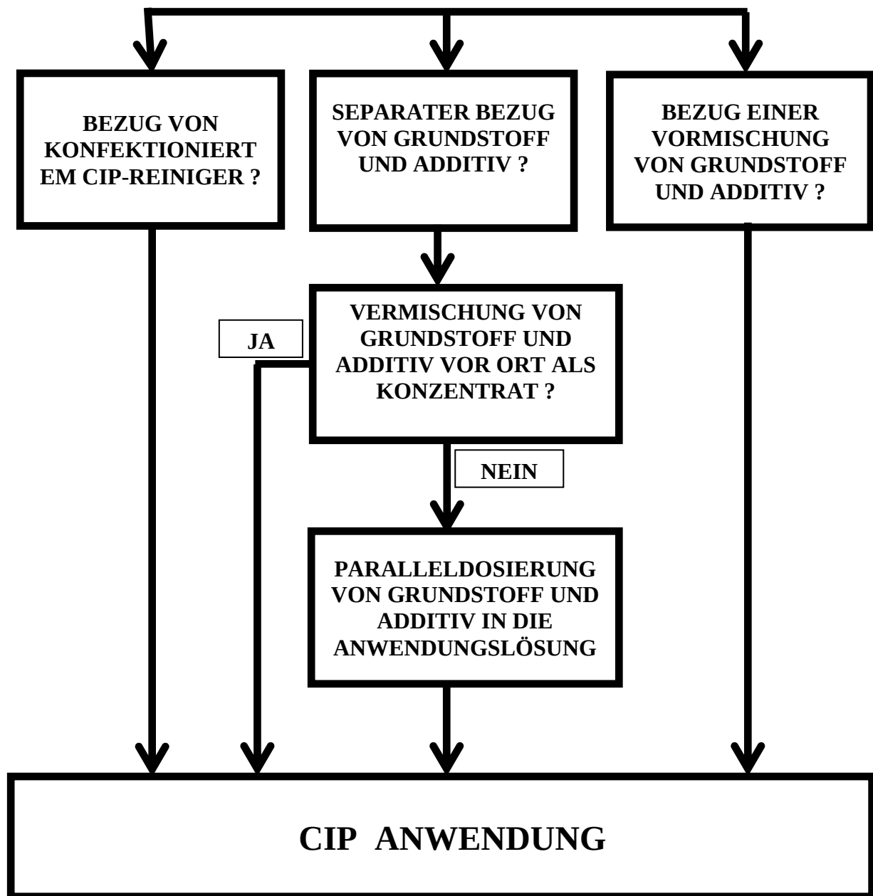
Abb. 1: Grundsätzliche Möglichkeiten der Chemikalienversorgung von CIP-Anlagen
